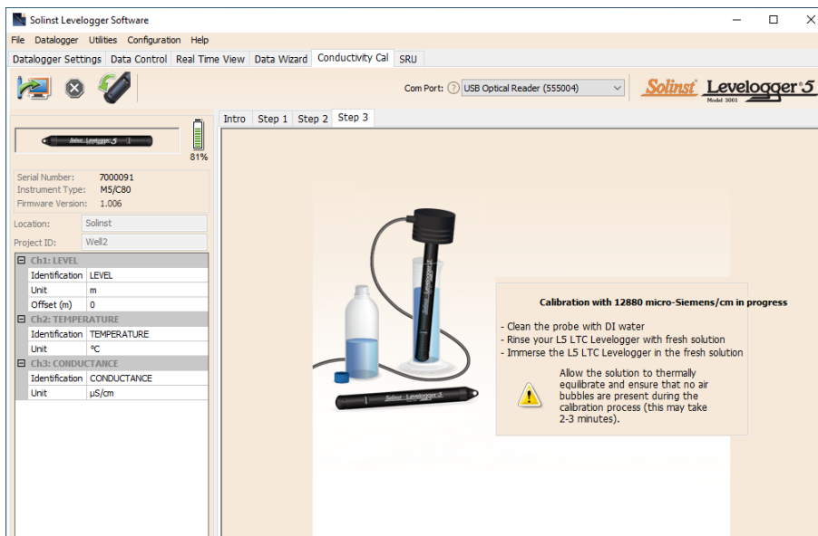
Figura 6-5 Paso 3 del Asistente de calibración de conductividad del Levelogger (ejemplo de la ventana de calibración con una solución de 12.880 µS/cm)
